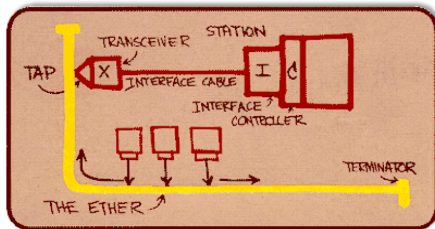
Esboço da Ethernet de Metcalfe
