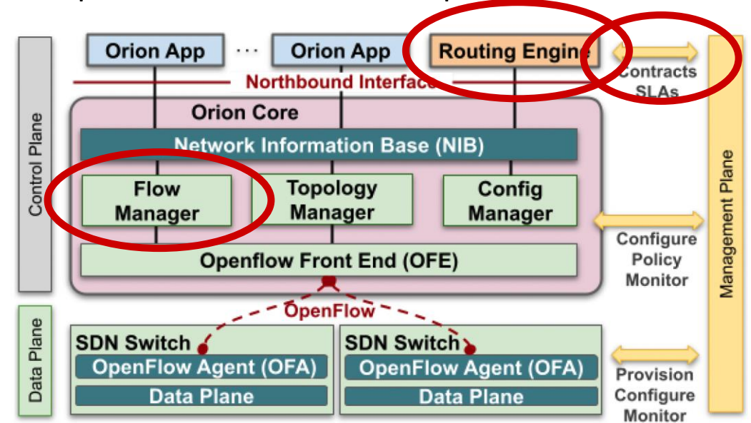
Arquitetura SDN do Orion e aplicativos de núcleo
